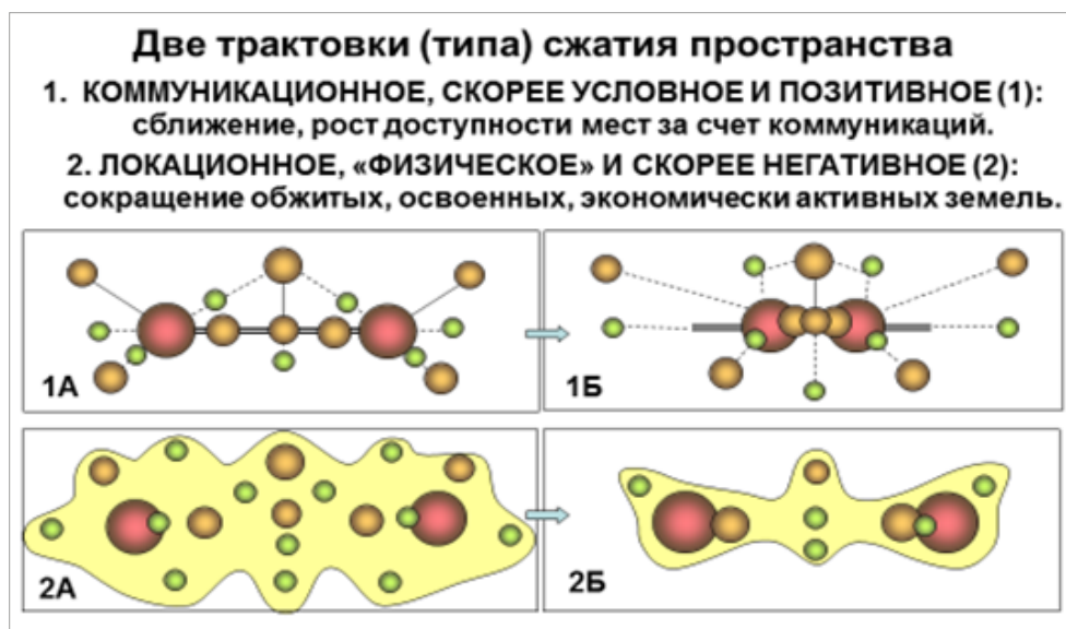
Рис. 20. Две трактовки сжатия пространства
